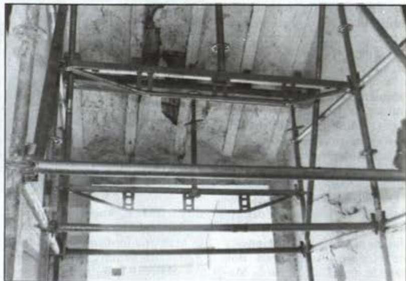
Un momento de la colocación de las talanqueras. A la derecha, un detalle del apuntalamiento en el que se aprecia el mal estado del tendido.
