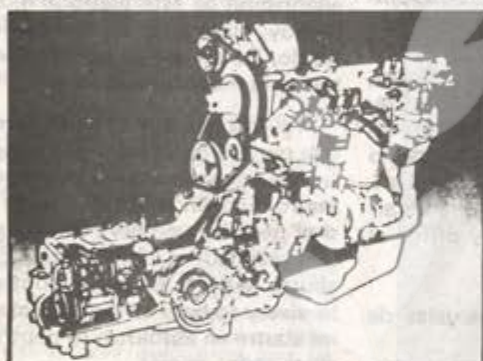
Motor: cigüeñal de 5 apoyos, camisas re-cambiables en cilindros, válvulas en cabeza.
