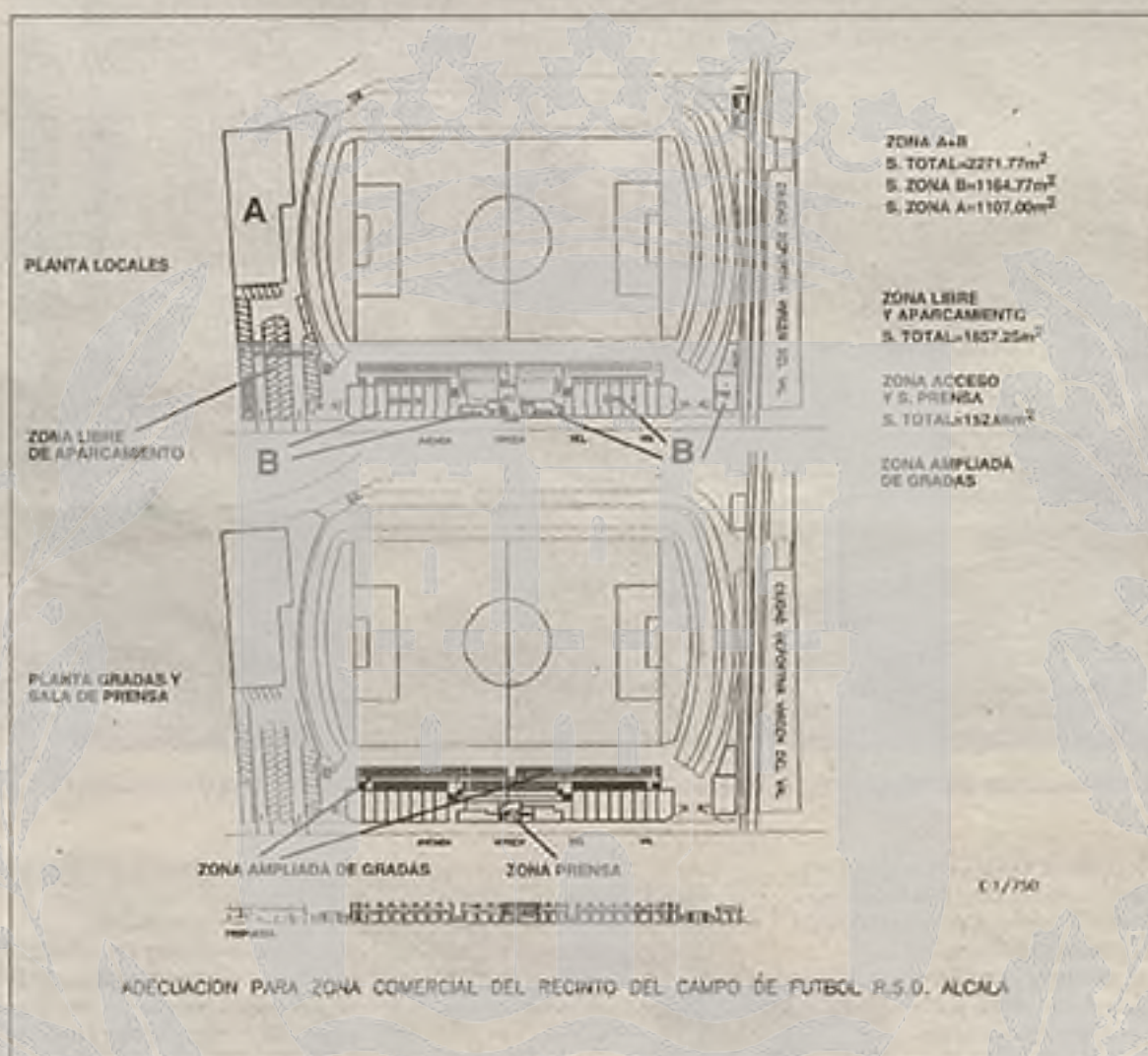
Dos de los planos que incluye el proyecto presentado por el Alcalá al Ayuntamiento
